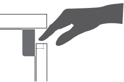
Gola piatta con tasca Flat groove with pocket
