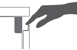
Gola con pesa maniglia “L” per gola piatta Flat “L” handle grip for flat groove
